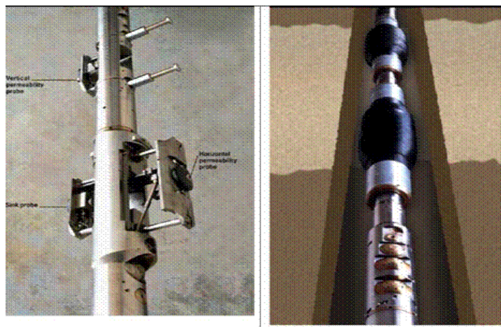
Рисунок 1 – Внешний вид прибора MDT: с прижимным зондом в варианте «прижимной зонд» (слева) и двухпакерная компоновка (справа)
