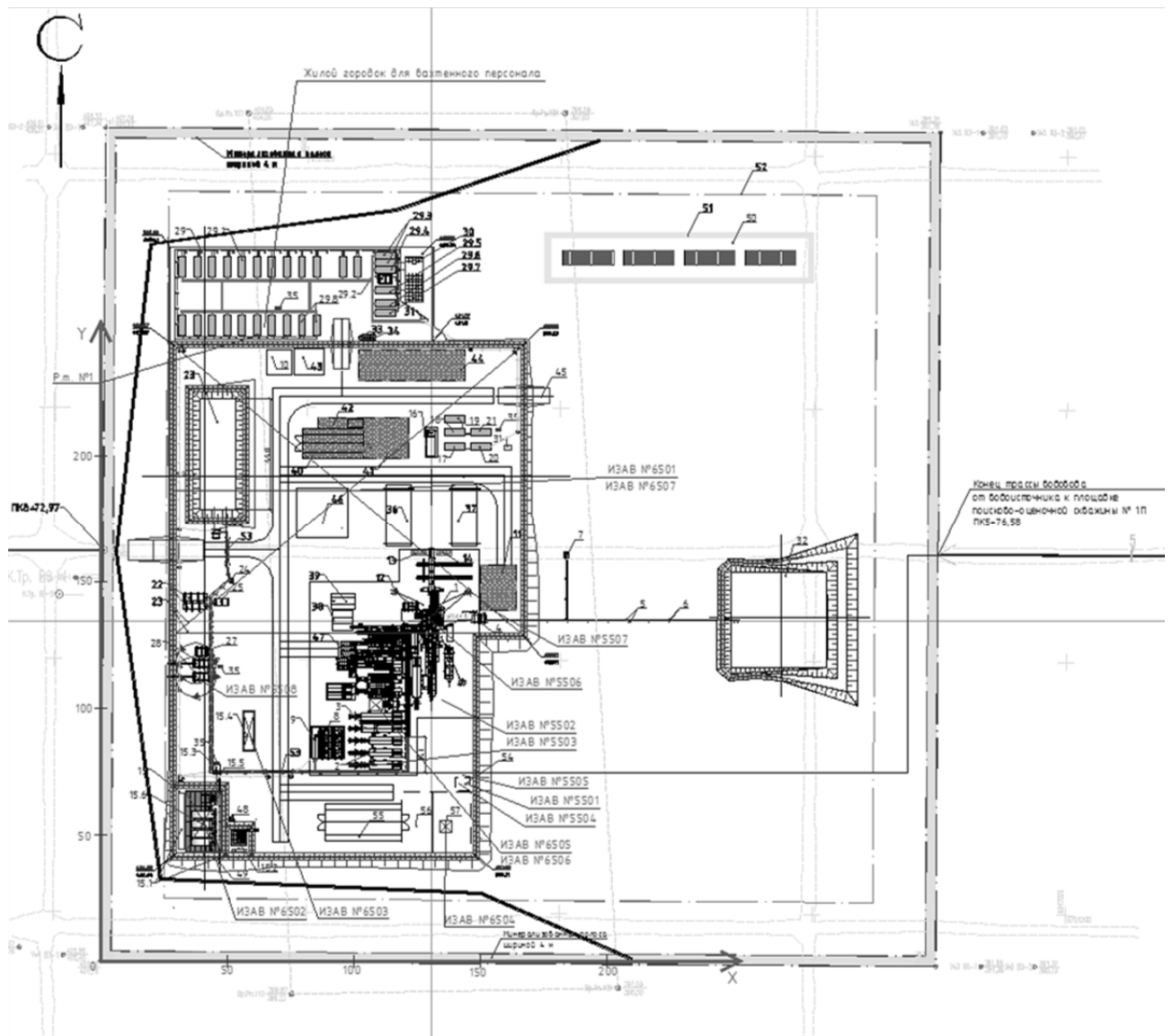
Рисунок 6.3.1 – Схема генплана скважины с расположением источников выбросов
