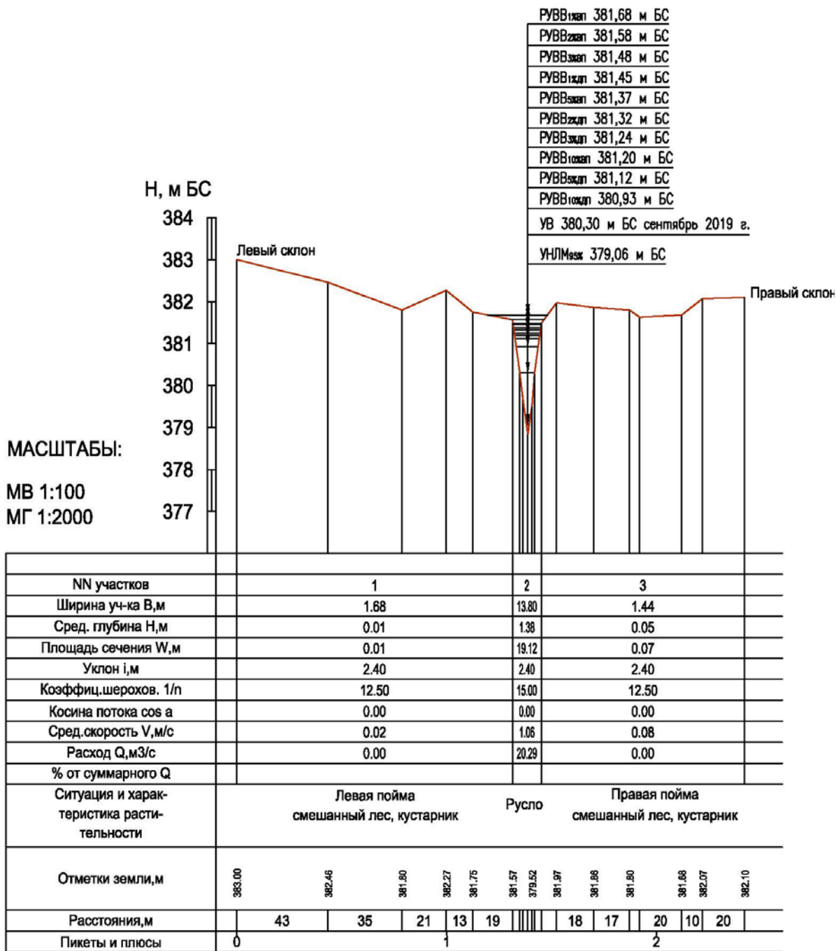
Рисунок 3.1 - Поперечный профиль долины руч. Куччугуй-Сюлдьюкээр
