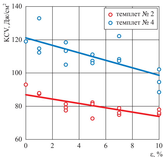
Рис. 8. Ударная вязкость в зависимости от степени предварительного деформирования стали 12ГСБ
