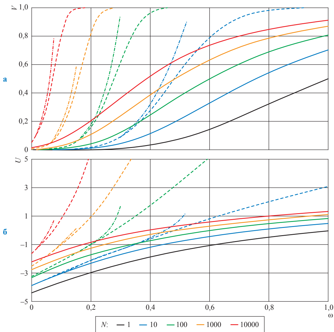
Рис. 2. Расчетная вероятность (а) и квантиль вероятности (б) отказа участка газопровода, состоящего из одинаковых дефектных труб в заданном количестве, в зависимости от уровня опасности дефектов
