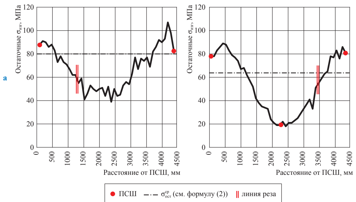
Рис. 9. Оценка остаточных нормальных напряжений при изгибе по периметрам одношовной (а) и двухшовной (б) труб
