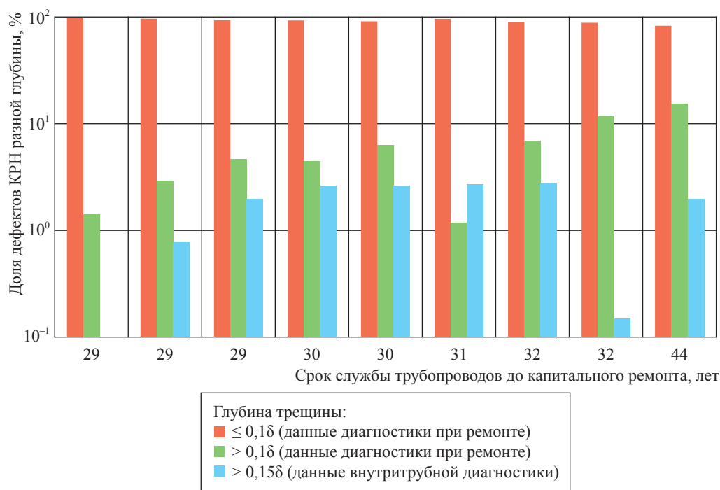
Рис. 1. Процентное отношение дефектов различной глубины к общему количеству дефектов КРН в зависимости от срока эксплуатации МГ
