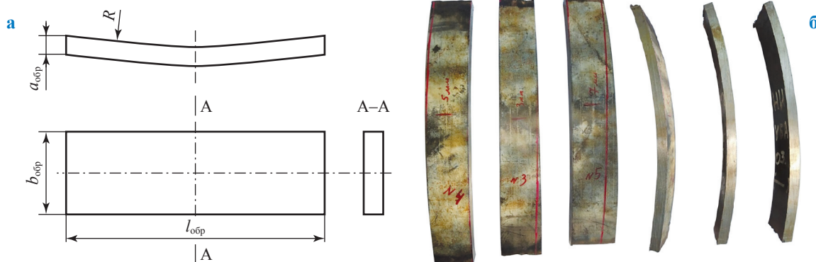
Рис. 1. Геометрия (а – схема; б – внешний вид) модельного образца после технологической обработки: R – радиус кривизны образца
