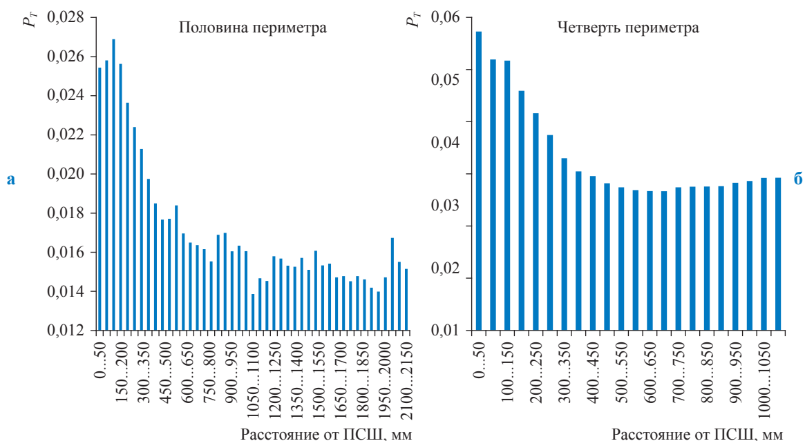
Рис. 7. Комплексный показатель вероятности распределения КРН в зависимости от расстояния до ПСШ для одношовных (а) и двухшовных (б) труб, по данным обследований в ходе КР
