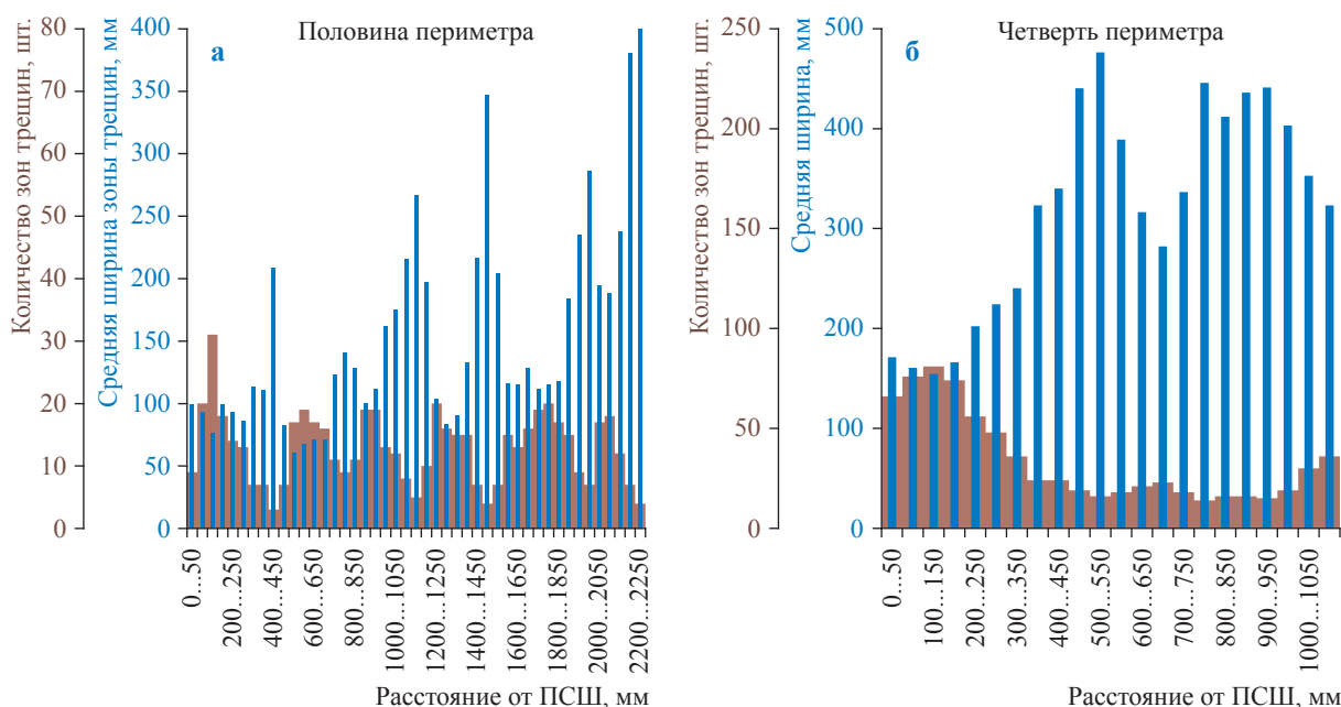
Рис. 5. Распределение ширины трещин КРН по расстоянию от шва для одношовных (а) и двухшовных (б) труб, составленное по данным ВТД
