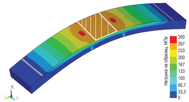
Рис. 6. Моделирование в программном комплексе ANSYS напряженного состояния в образце при усилки на опорах 19,7 кН
