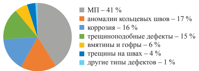
Рис. 2. Процентное соотношение недопустимых дефектов по результатам внутритрубной диагностики в 2018–2020 гг.
