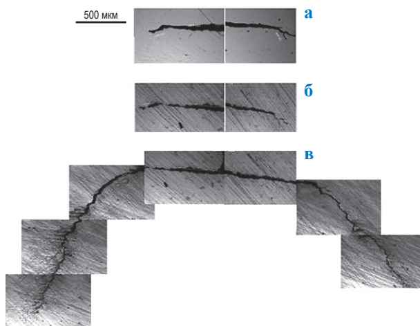
Рис. 10. Трансформация вершины естественной КРН-трещины в образце № 1 на разных этапах испытаний: а – трещина в исходном состоянии; б – после 2000 циклов; в – после 4000 циклов
