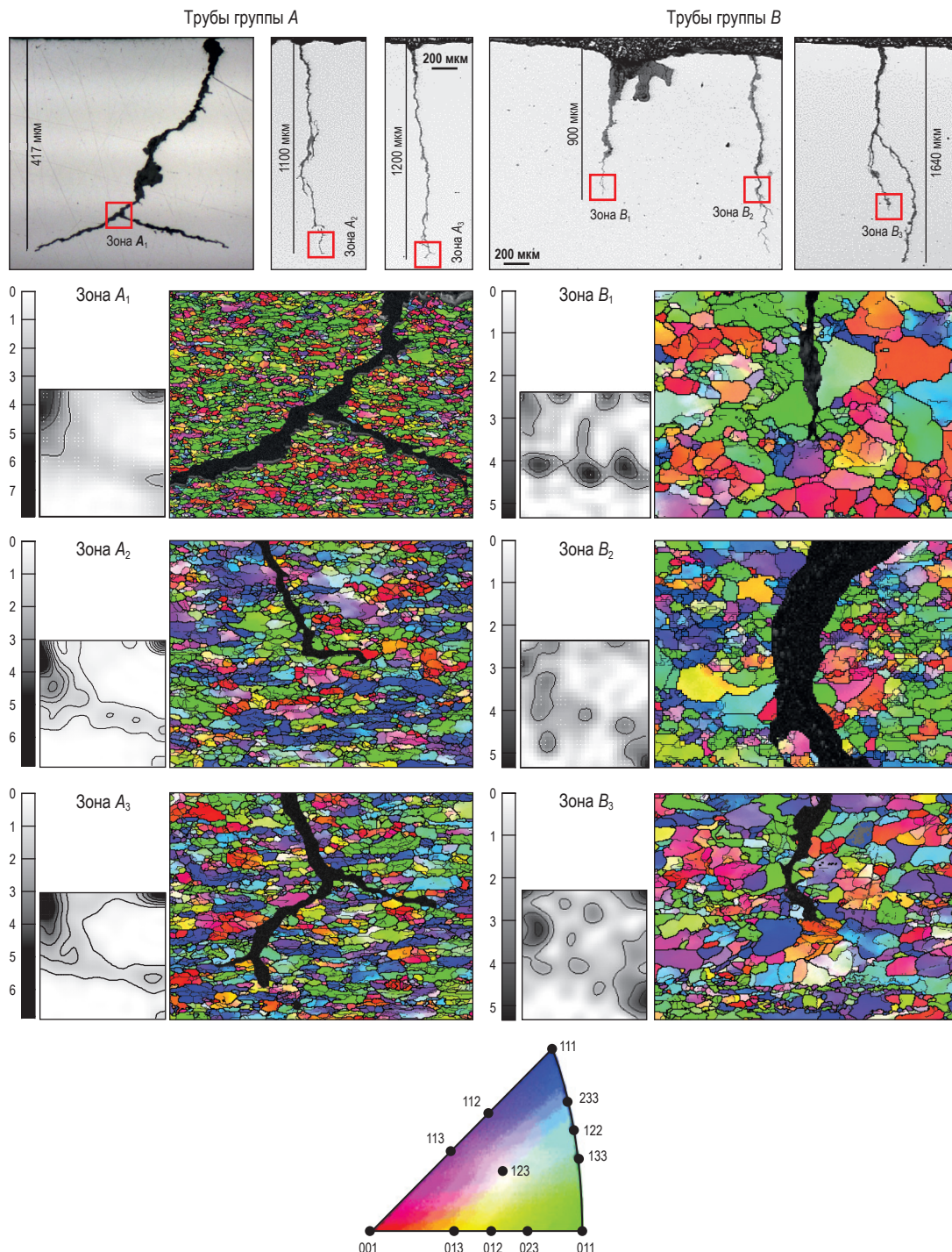
Рис. 5. EBSD-карты ориентаций зерен в поверхностных слоях труб и соответствующие им сечения ФПО при \varphi_2 = 45^\circ : цветами RGB-палитры представлены зерна, имеющие различную кристаллографическую ориентацию, определенную в пределах элементарного стереографического треугольника для кубических материалов
