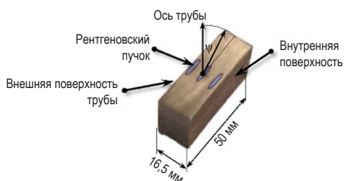
Рис. 2. Схема измерения остаточных упругих деформаций в образцах труб МГ рентгеновским методом: \psi – угол наклона образца
