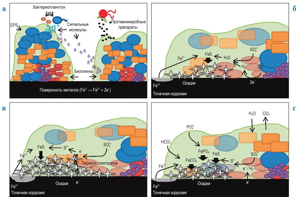
Рис. 2. Схема биоэлектрохимических процессов, протекающих на поверхности стали [32]: а – биопленка на поверхности металла, продуцирующая сигнальные молекулы и противомикробные препараты; б – химическая коррозия, вызванная сульфатредуцирующими бактериями (СРБ); в – электрическая микробиологическая коррозия, вызванная СРБ; г – многослойная биопленка, приводящая к образованию нескольких различных осадков
